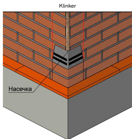
Рис. 21. Монтаж последующих угловых элементов.
